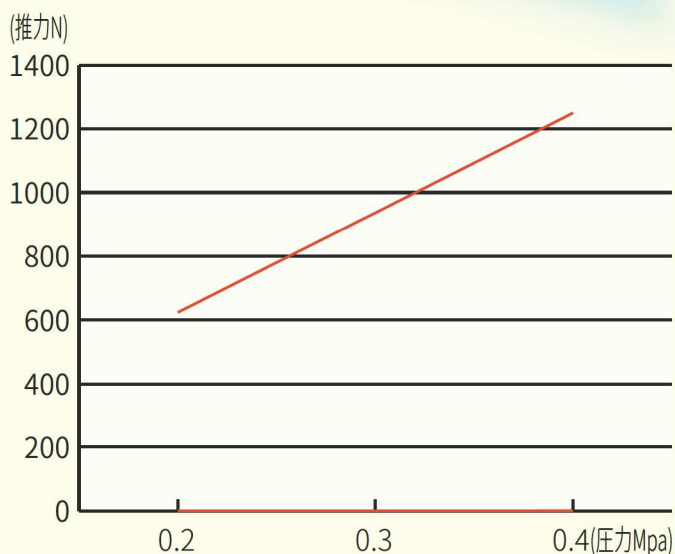
■カシメヘッド推力表
